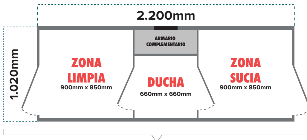
Plano a escala de U.M.D. Modelo: 220/10 S.D.
